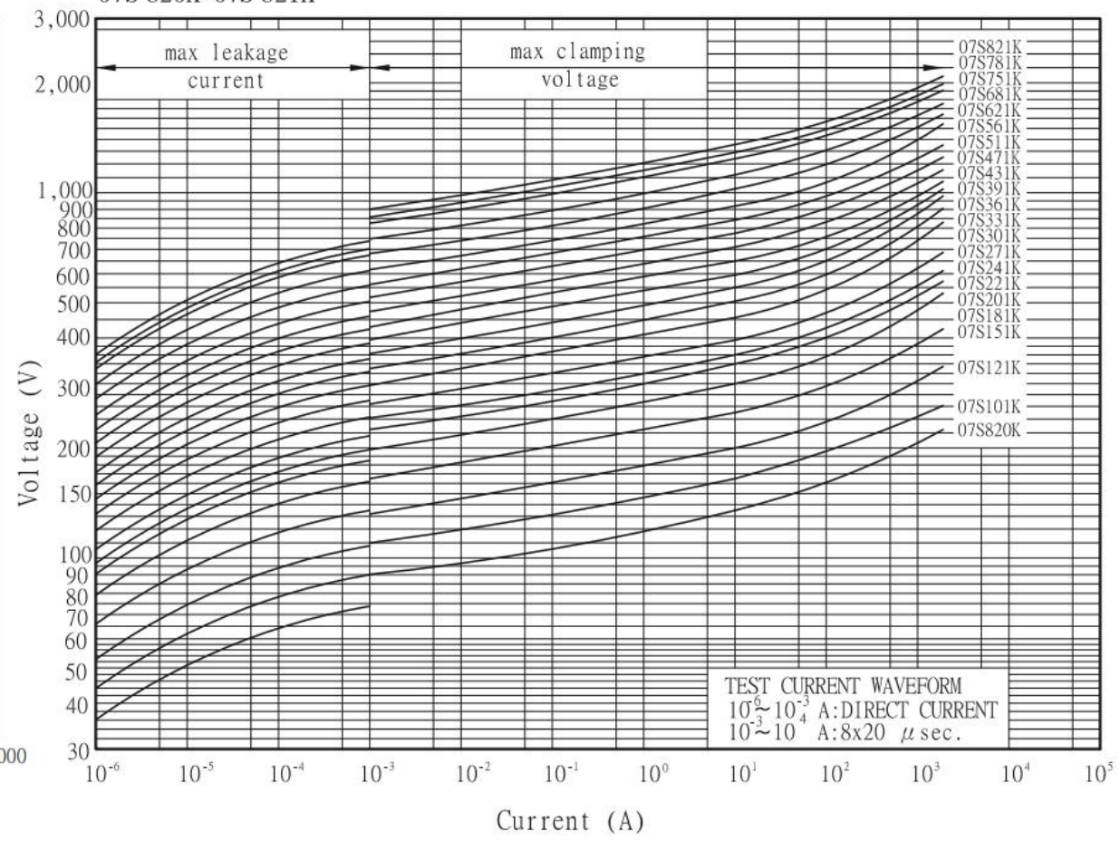
07S 820K~07S 821K
