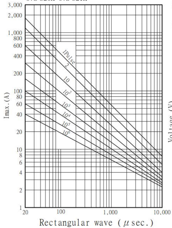
07S 820K~07S 821K
