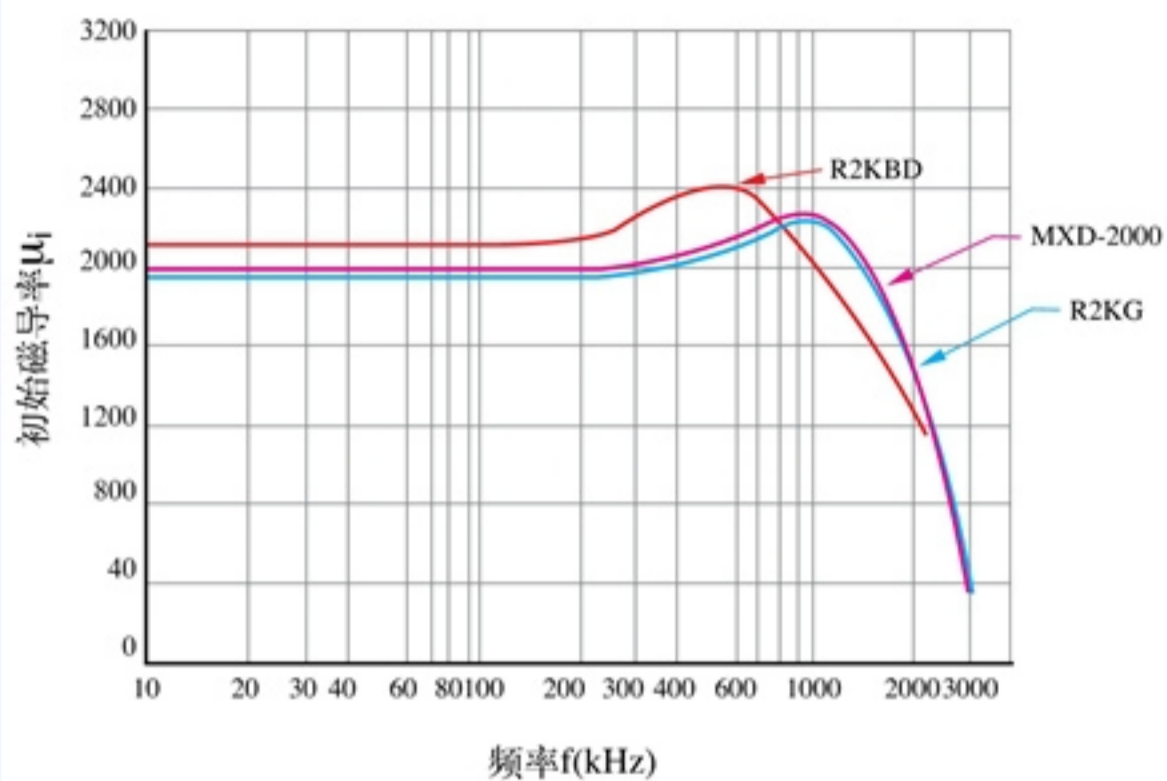
频率曲线( \mu_i -f)
