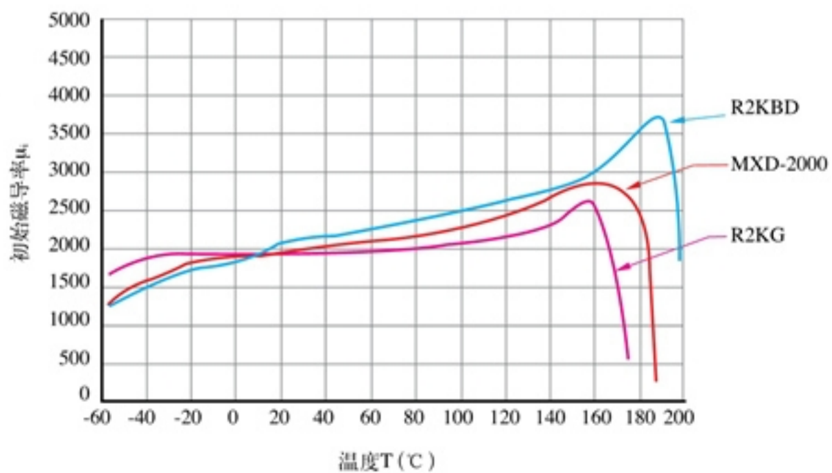
初始磁导率温度曲线( \mu_i -T)
