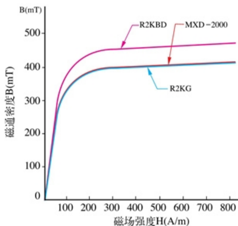
磁化曲线(B-H)
