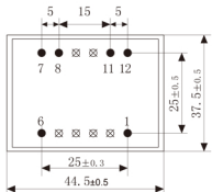
底视图
