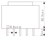
主视图
