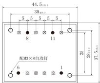
底视图
