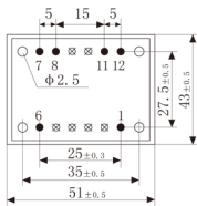
底视图
