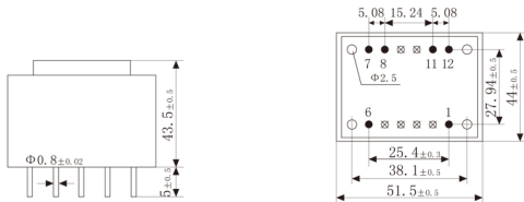
主视图
