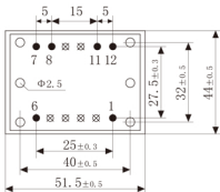
底视图
