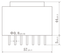
主视图
