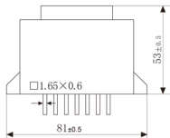
主视图
