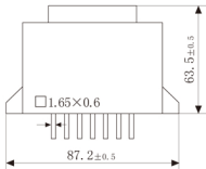
主视图
