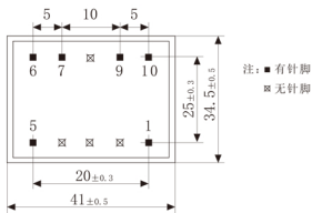
底视图(环氧面)
