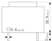
主视图
