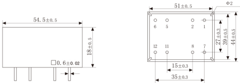
主视图
