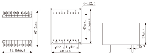
顶视图
