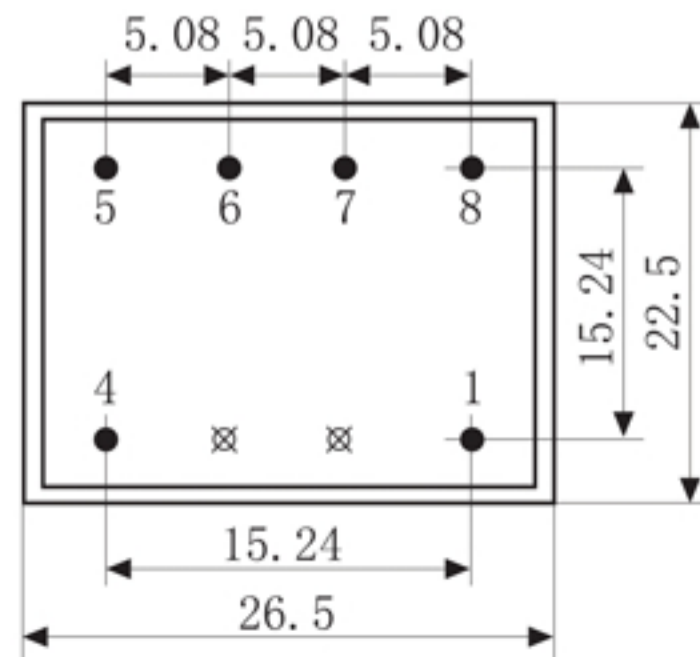
底视图
