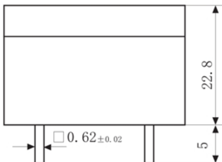
主视图
