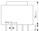
主视图
