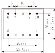
底视图
