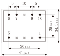
底视图
