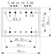
底视图
