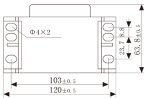
顶视图
