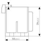
侧视图
