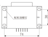
顶视图
