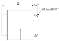
侧视图
