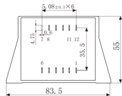
主视图
