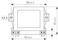
顶视图
