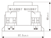
主视图
