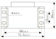
顶视图
