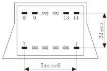
主视图
