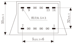
主视图
