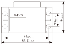
顶视图
