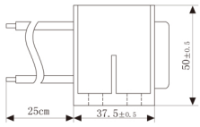
侧视图
