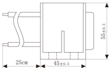
侧视图
