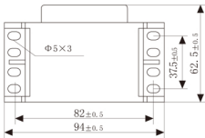
顶视图
