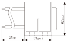
侧视图
