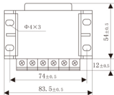
顶视图
