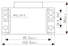
顶视图
