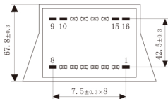
主视图
