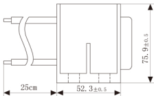
侧视图
