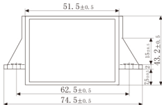
侧视图
