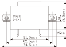
顶视图
