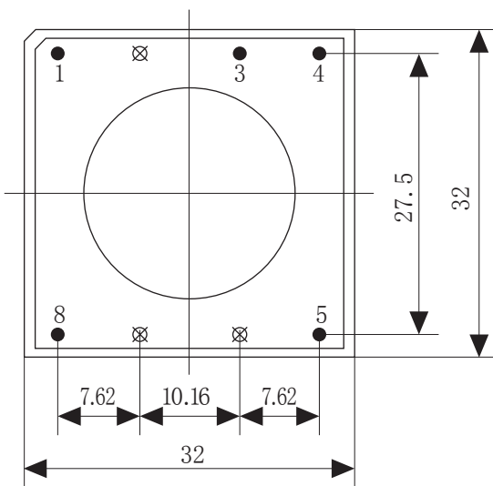
底视图
