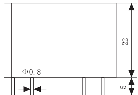
主视图
