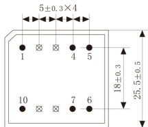
底视图
