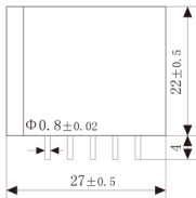
主视图
