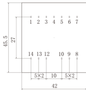
底视图
