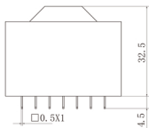
主视图
