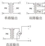
原理图
