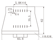
背视图(P型焊片引出方式)
