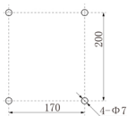
固定孔尺寸图
