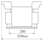
侧视图
