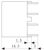
侧视图
