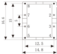
底视图
