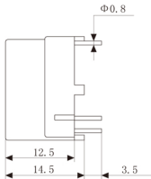
侧视图
