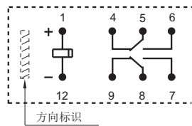
单稳态
